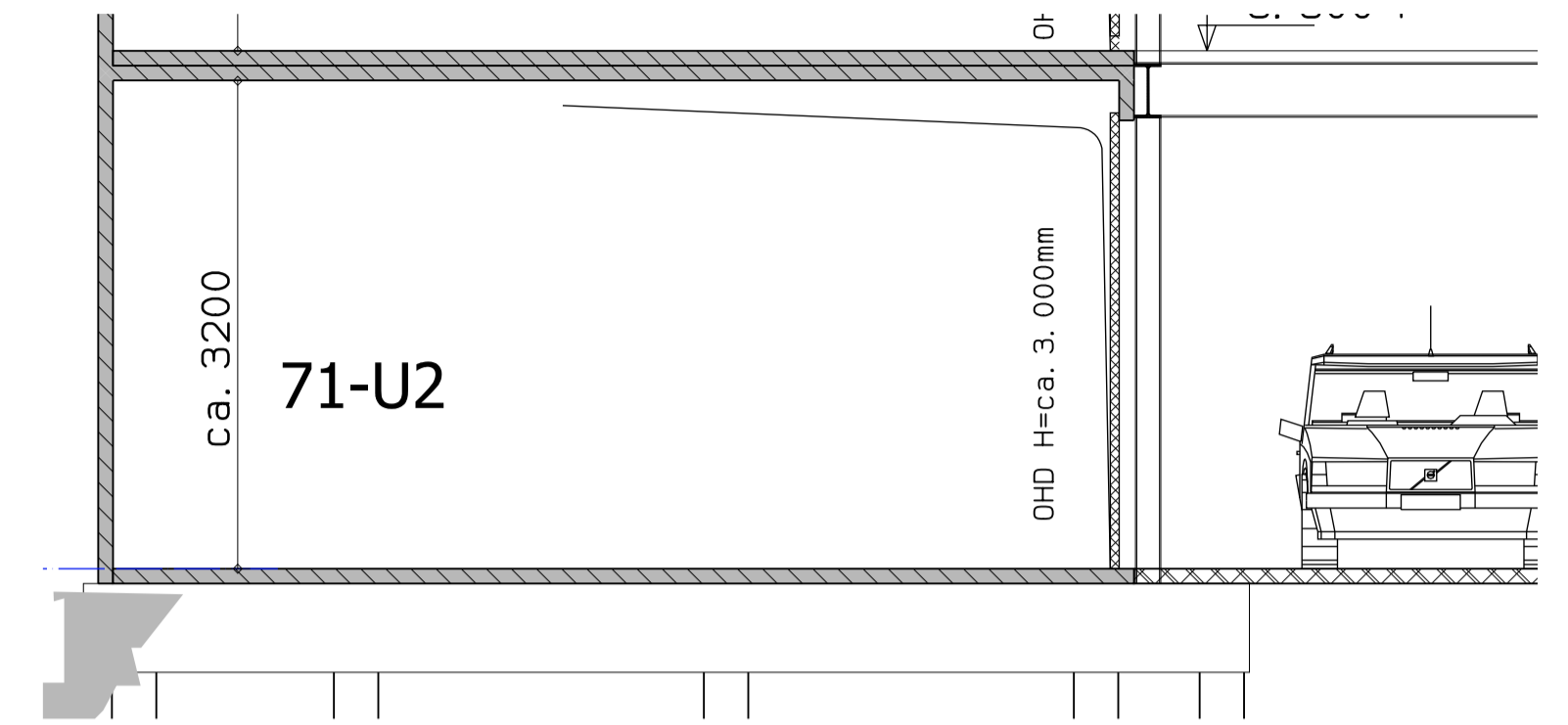
DWARSDOORSNEDE BOUWNUMMER BOX 71-U2
