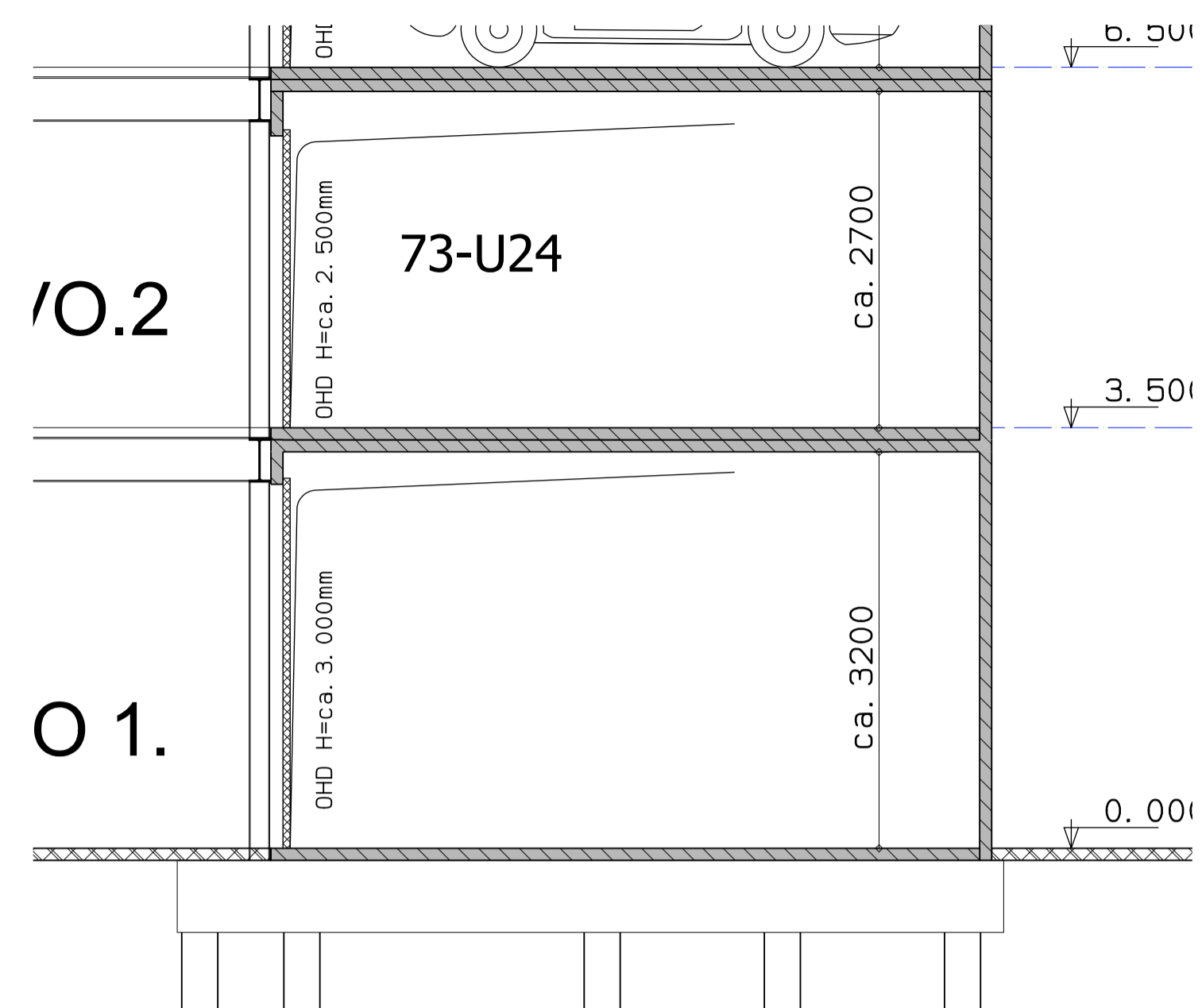
DWARSDOORSNEDE BOUWNUMMER BOX 73-U24
