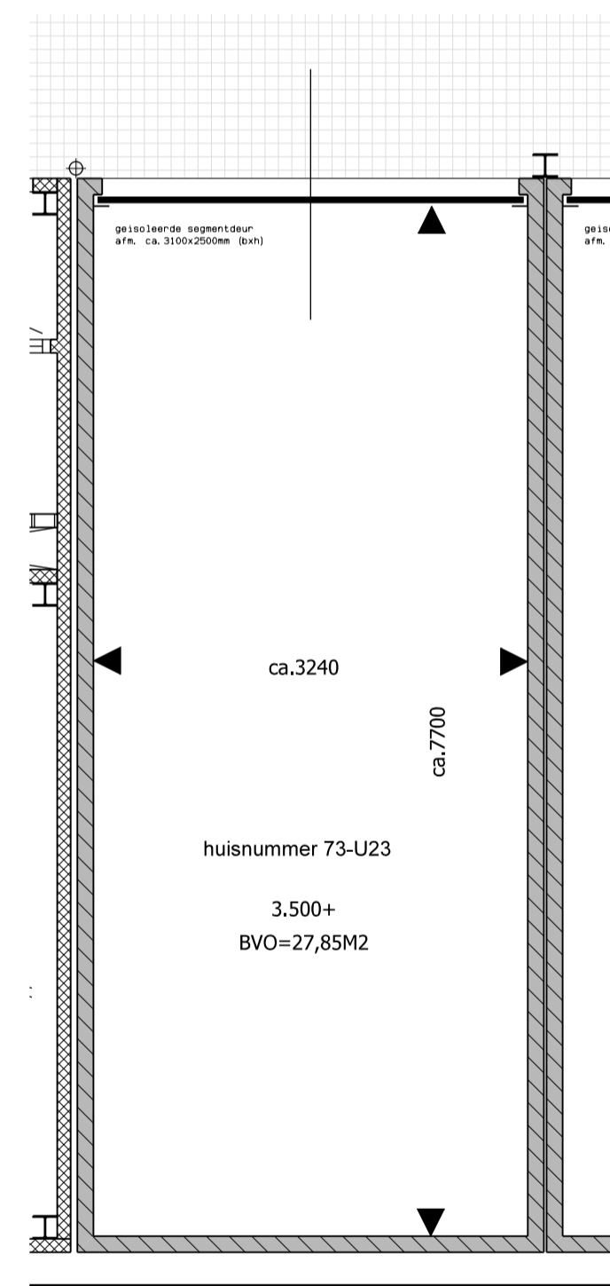
PLATTEGROND VERDIEPING BOUWNUMMER BOX 73-U23
