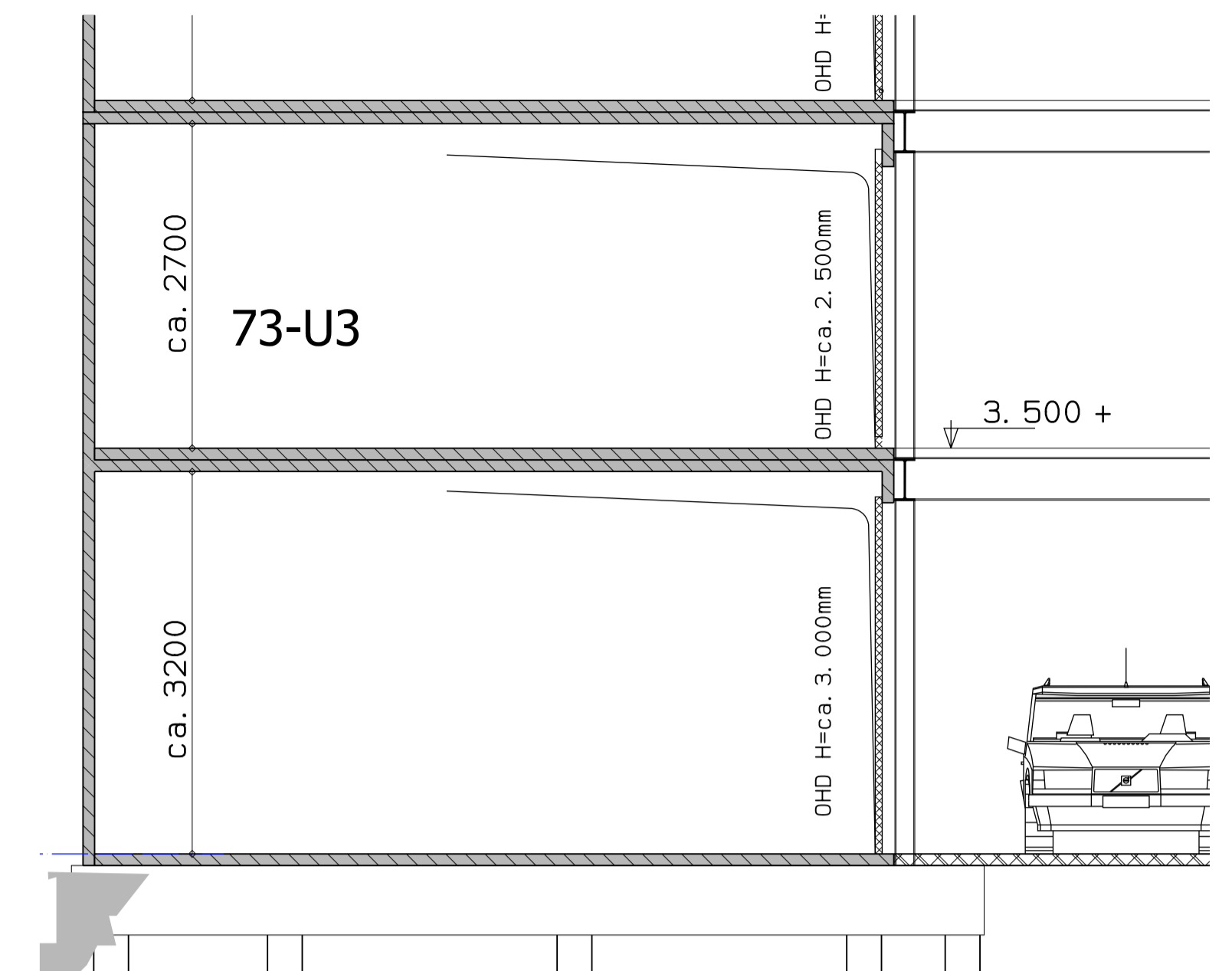
DWARSDOORSNEDE BOUWNUMMER BOX 73-U3
