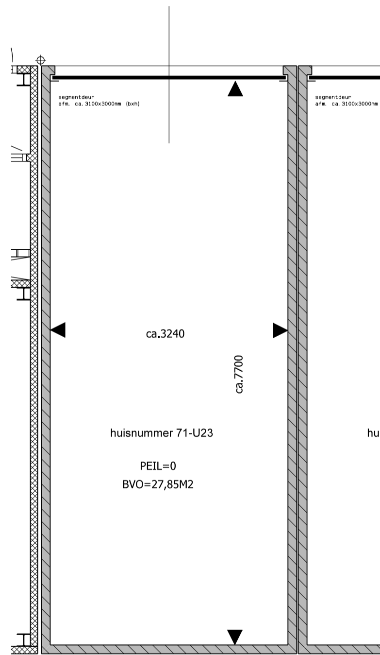
PLATTEGROND BEGANEGROUND BOUWNUMMER BOX 71-U23
