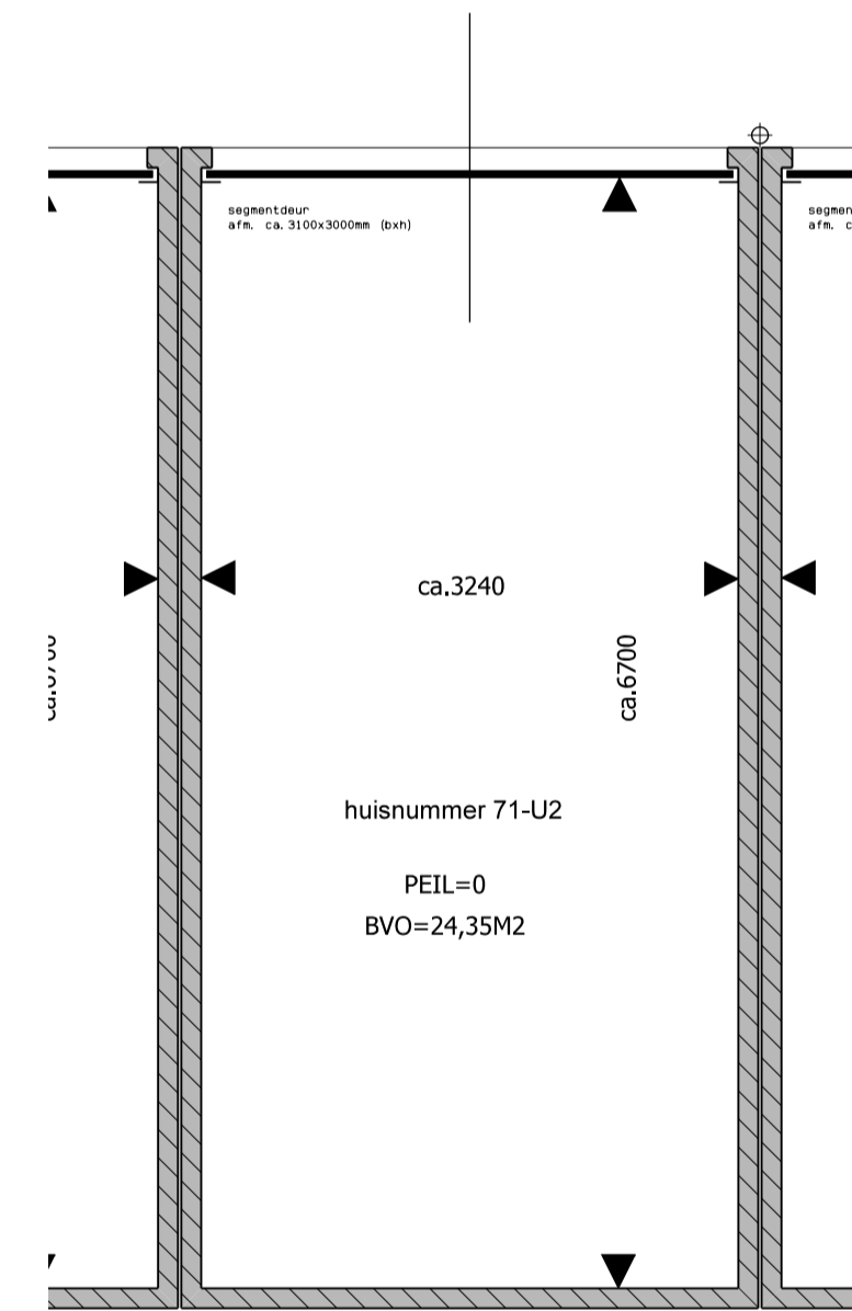
PLATTEGROND BEGANEGROUND BOUWNUMMER BOX 71-U2
