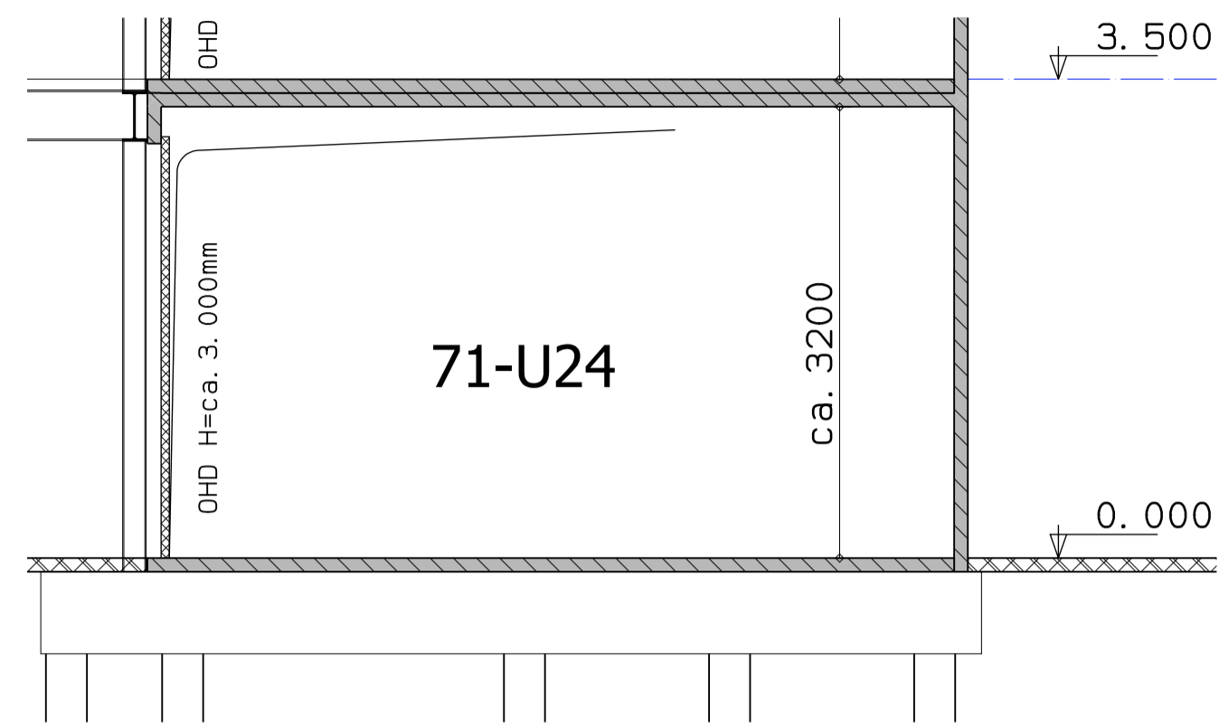
DWARSDOORSNEDE BOUWNUMMER BOX 71-U24
