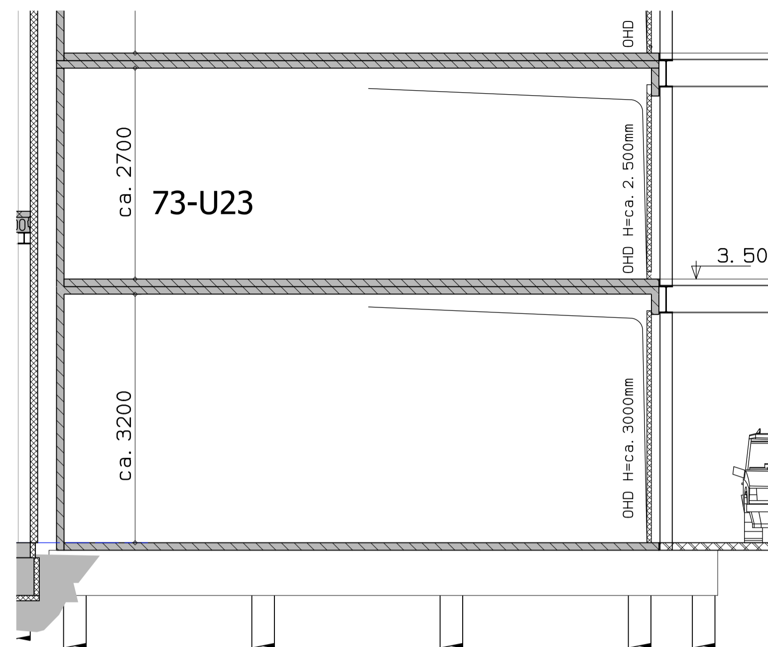
DWARSDOORSNEDE BOUWNUMMER BOX 73-U23
