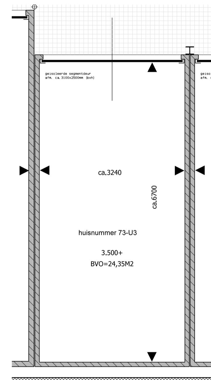
PLATTEGROND VERDIEPING BOUWNUMMER BOX 73-U3
