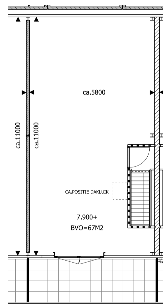
PLATTEGROND 2E VERDIEPING UNIT BOUWNUMMER 61
