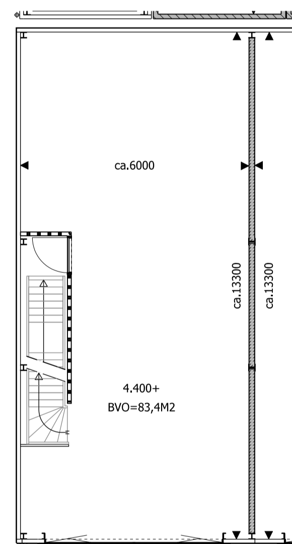
PLATTEGROND 1E VERDIEPING UNIT BOUWNUMMER 35
