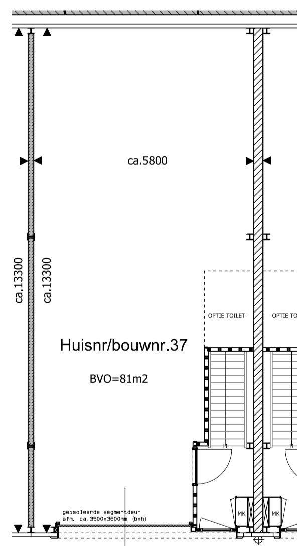
PLATTEGROND BEGANEGROND UNIT BOUWNUMMER 37t/m59
