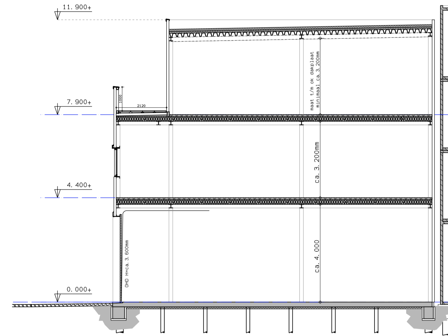
DWARSDOORSNEDE UNIT BOUWNUMMER 37t/m59
