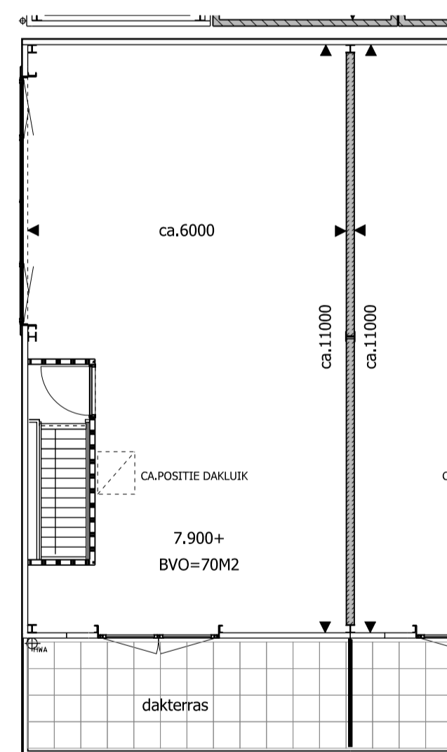
PLATTEGROND 2E VERDIEPING UNIT BOUWNUMMER 35
