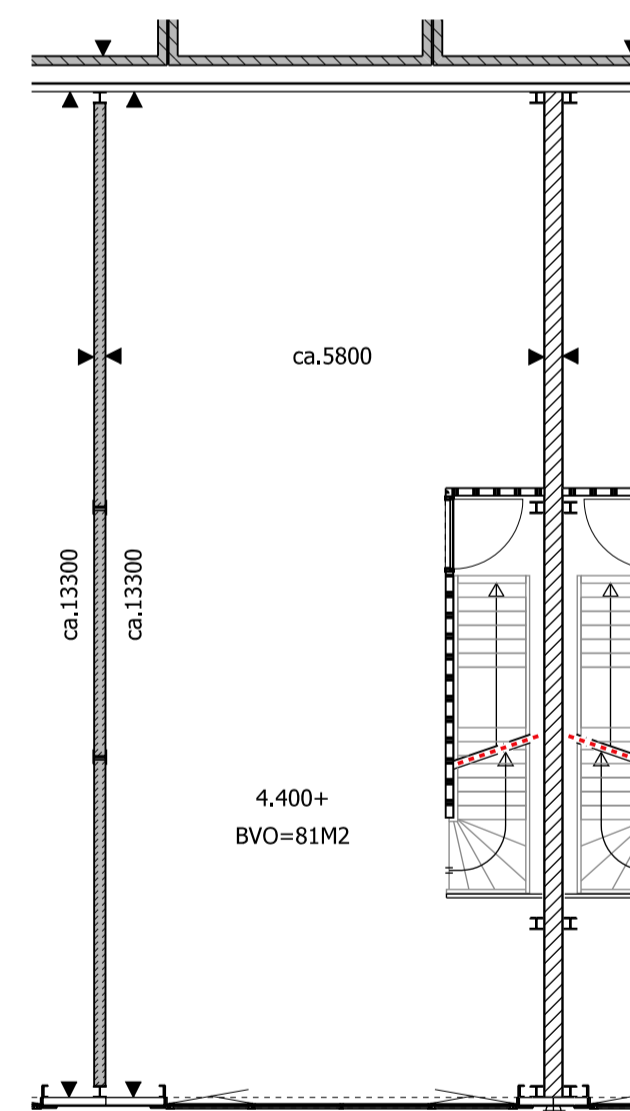
PLATTEGROND 1E VERDIEPING UNIT BOUWNUMMER 37t/m59
