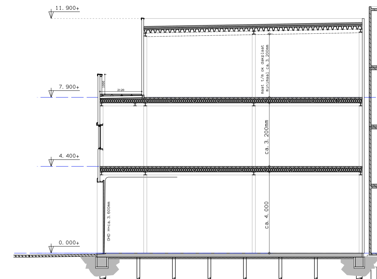
DWARSDOORSNEDE UNIT BOUWNUMMER 35
