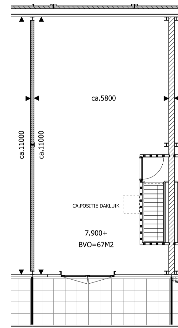
PLATTEGROND 2E VERDIEPING UNIT BOUWNUMMER 37t/m59
