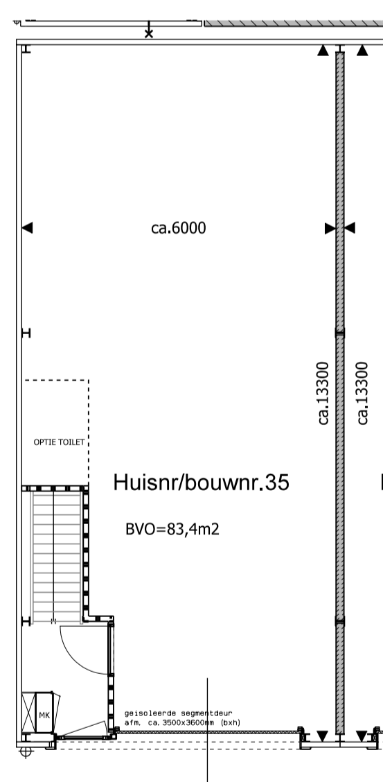
PLATTEGROND BEGANEGROND UNIT BOUWNUMMER 35
