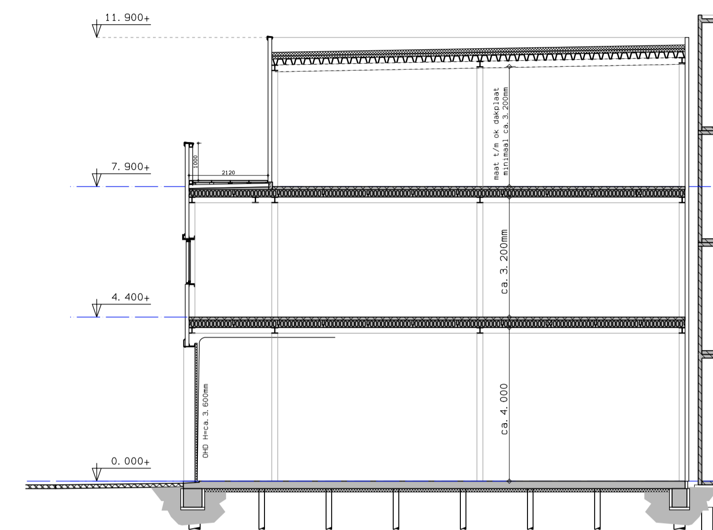
DWARSDOORSNEDE UNIT BOUWNUMMER 61
