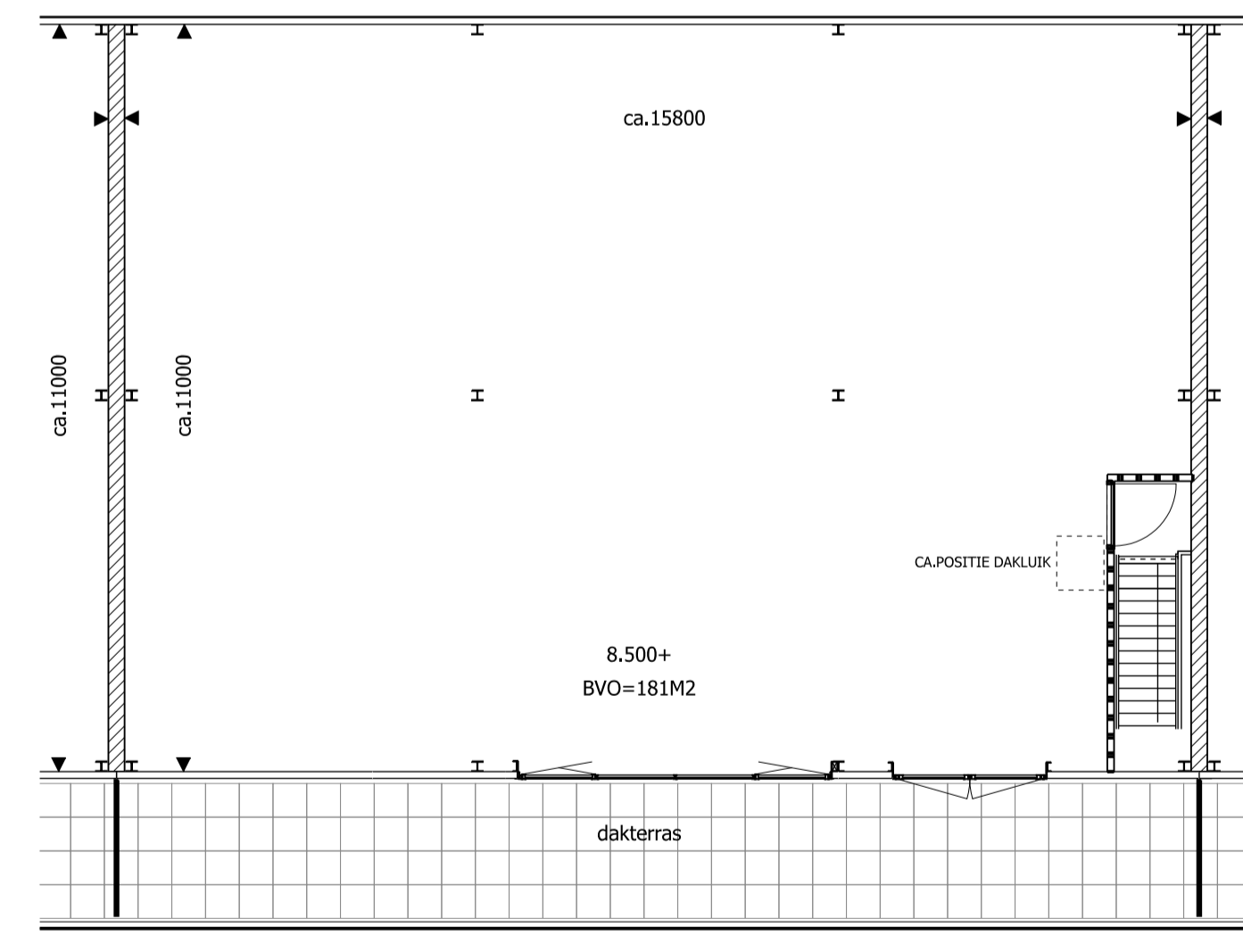
2e VERDIEPING UNIT BOUWNUMMER 29
