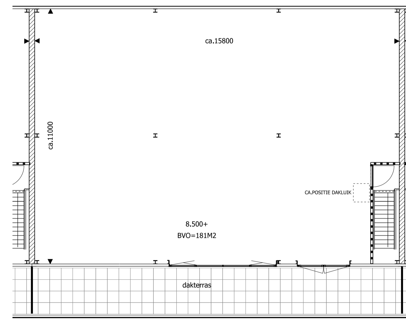
2e VERDIEPING UNIT BOUWNUMMER 31
