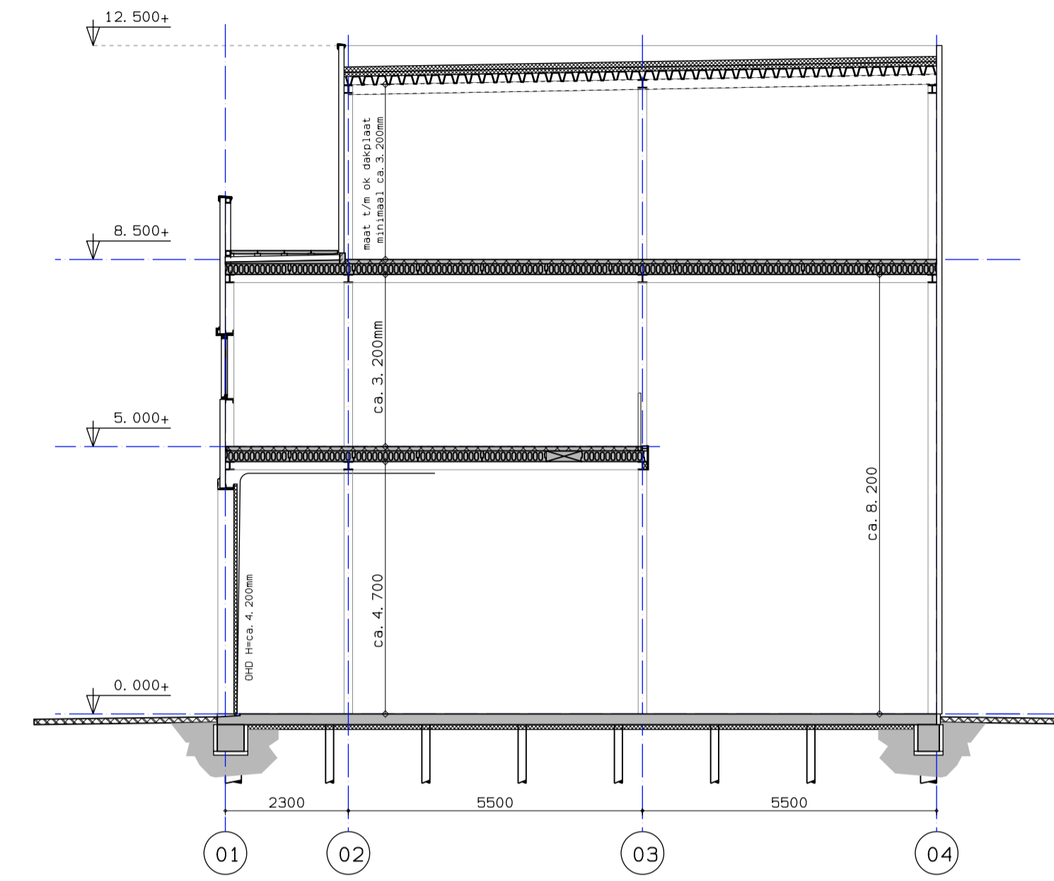
DWARSDOORSNEDE UNIT BOUWNUMMER 33
