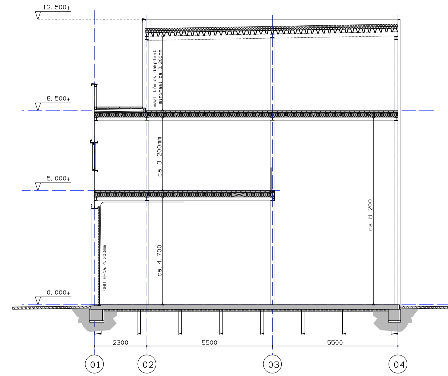
DWARSDOORSNEDE UNIT BOUWNUMMER 27
