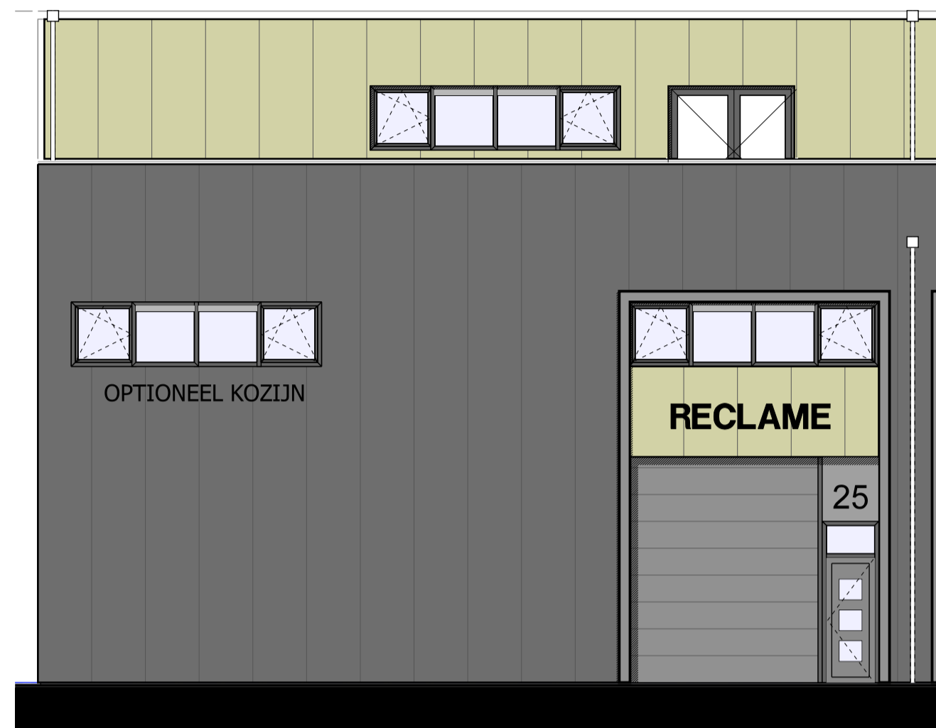
VOORAANZICHT UNIT BOUWNUMMER 25
