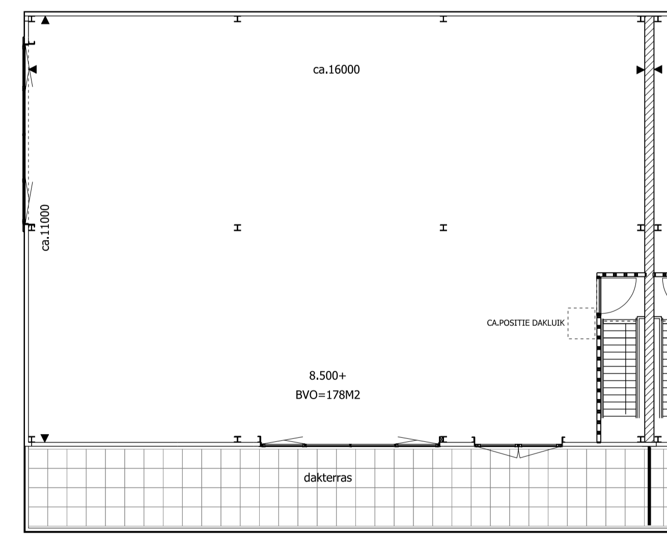
2e VERDIEPING UNIT BOUWNUMMER 25
