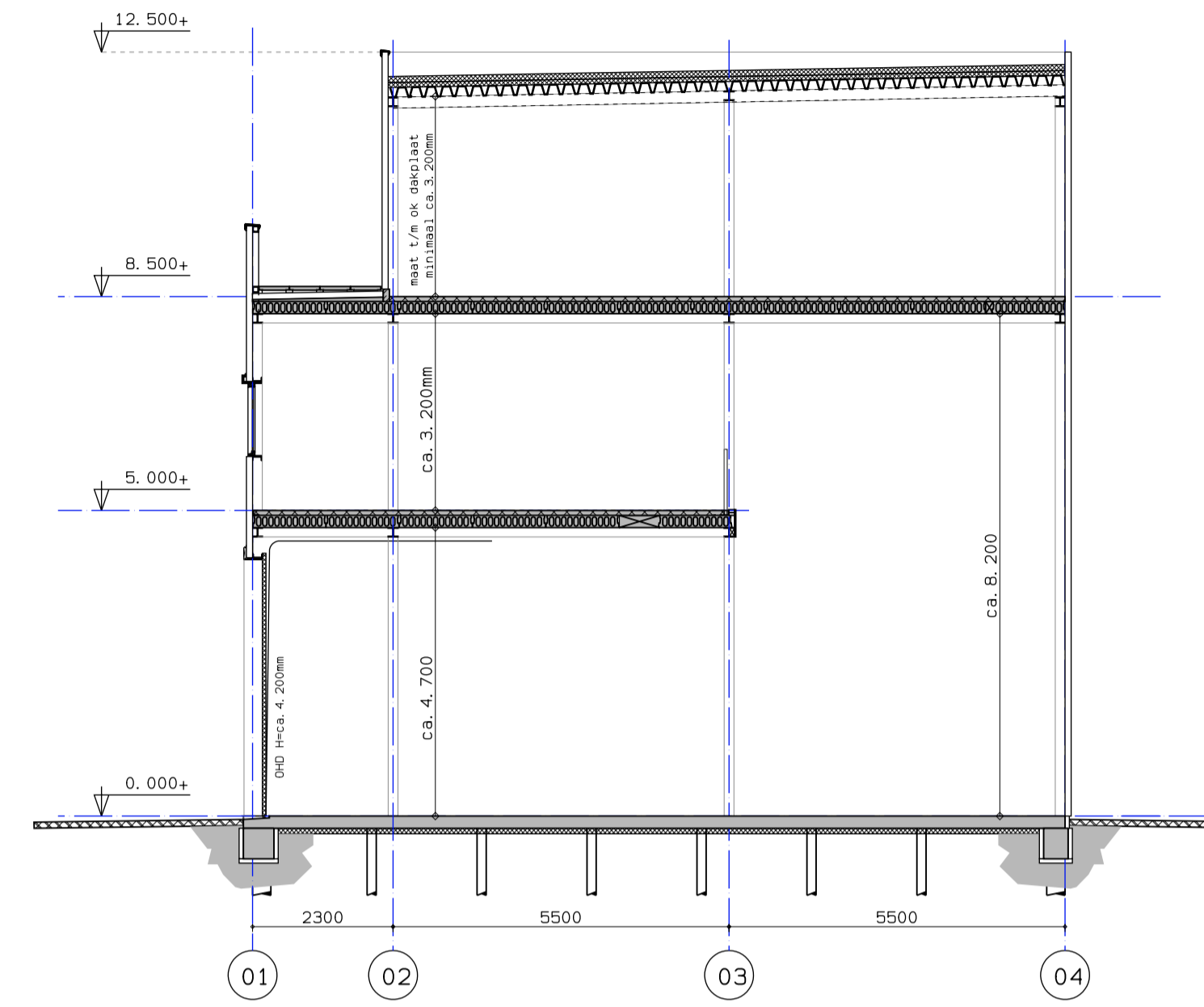
DWARSDOORSNEDE UNIT BOUWNUMMER 31
