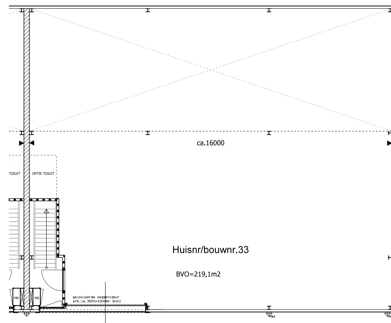
PLATTEGROND UNIT BOUWNUMMER 33
