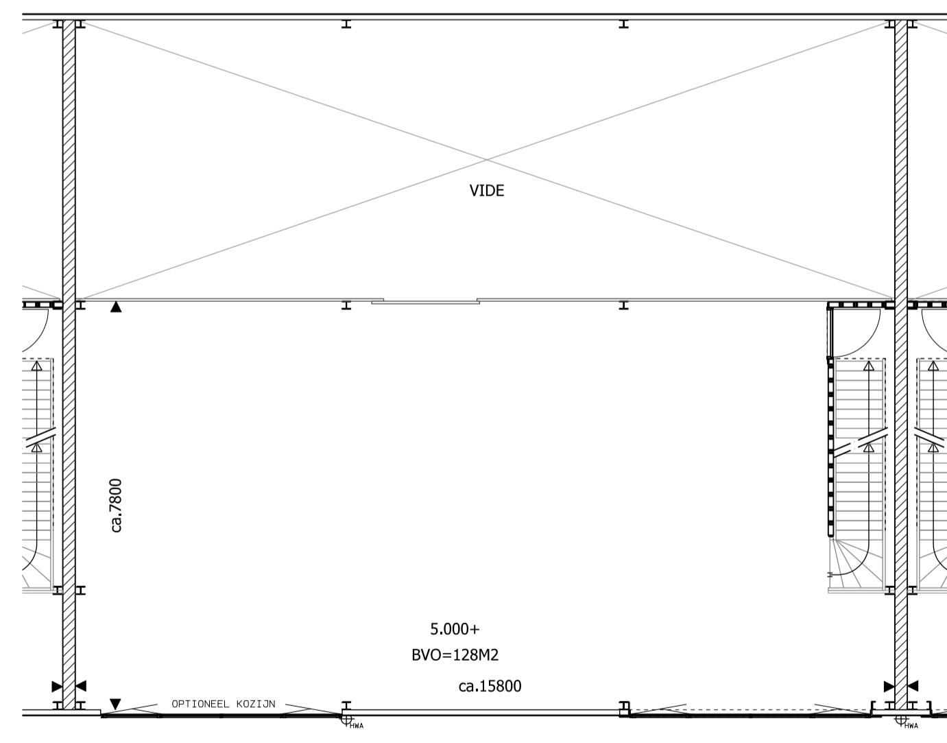
1e VERDIEPING UNIT BOUWNUMMER 31
