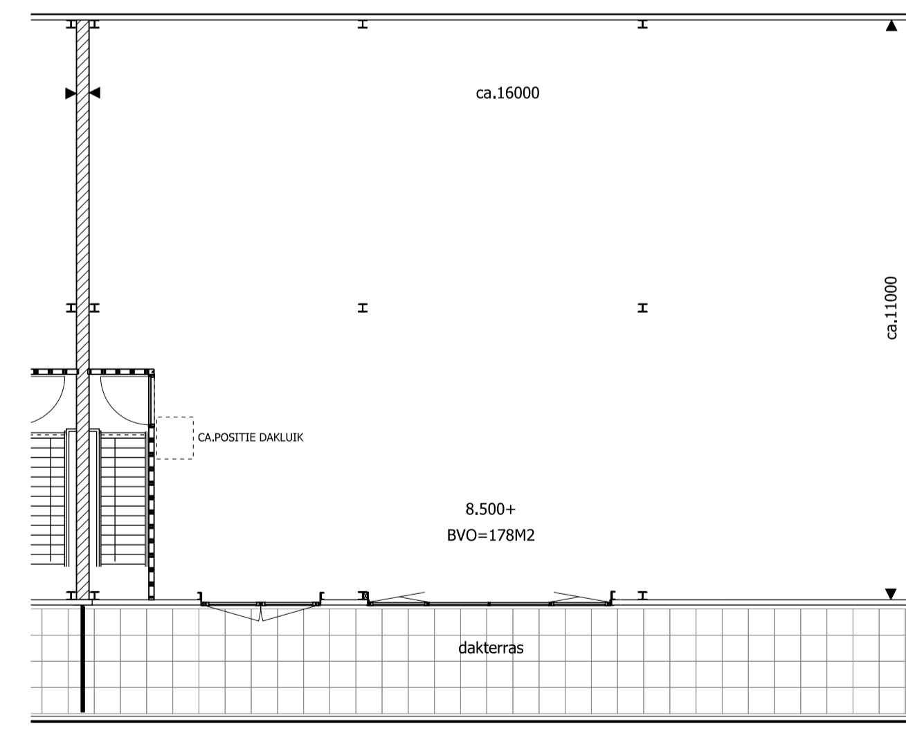
2e VERDIEPING UNIT BOUWNUMMER 33
