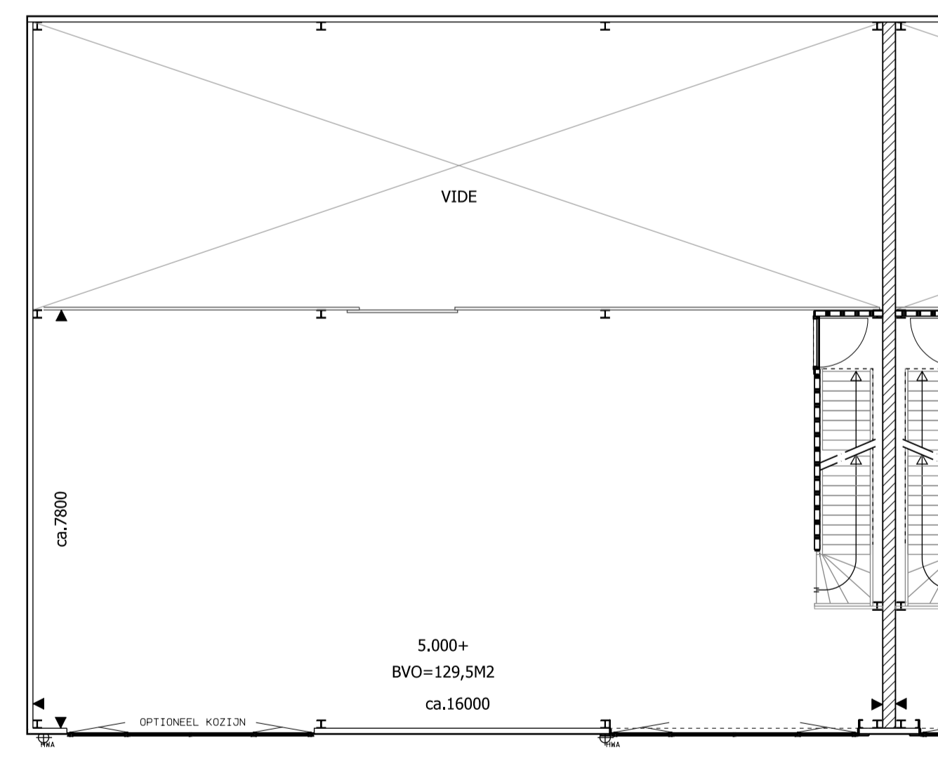
1e VERDIEPING UNIT BOUWNUMMER 25
