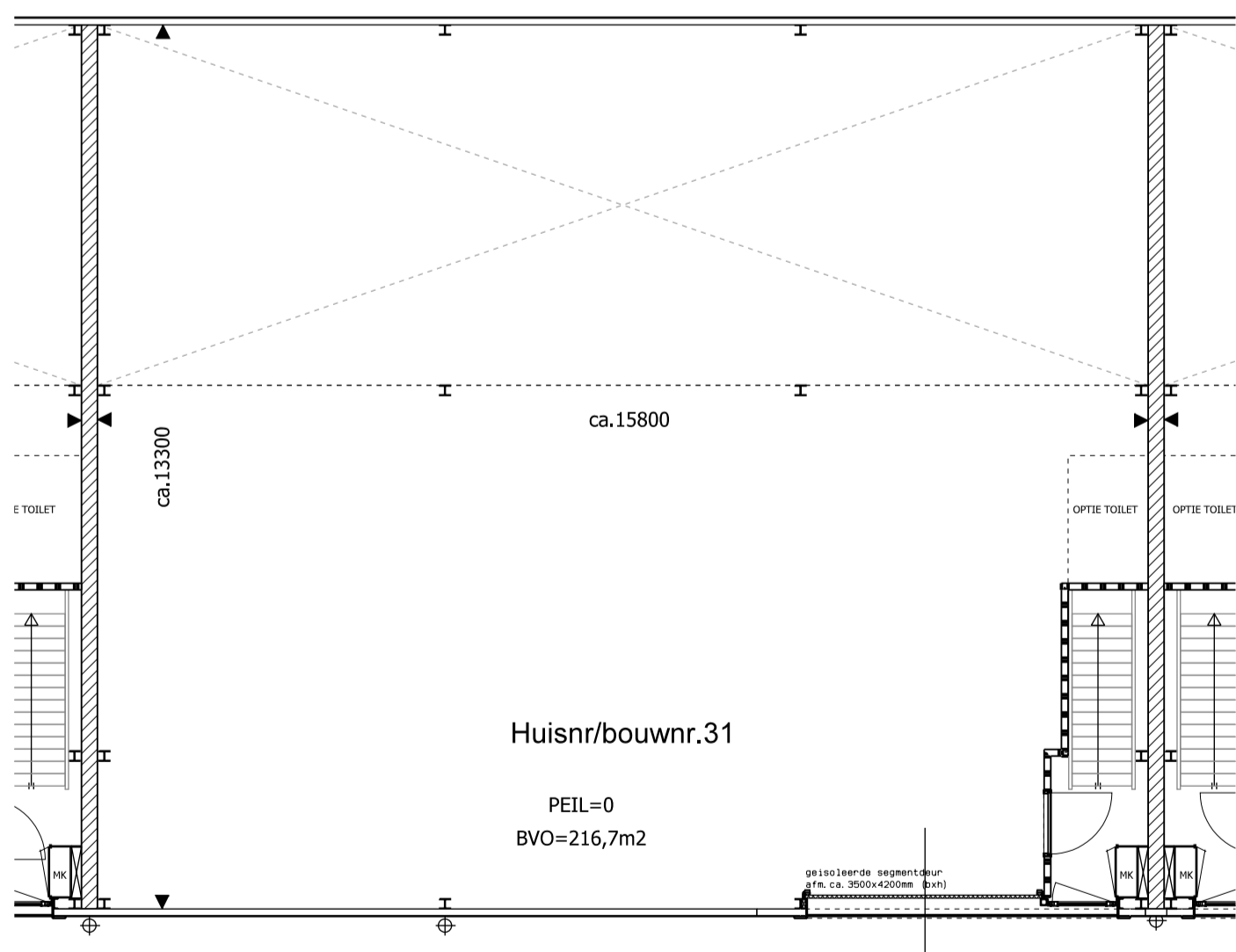
PLATTEGROND UNIT BOUWNUMMER 31
