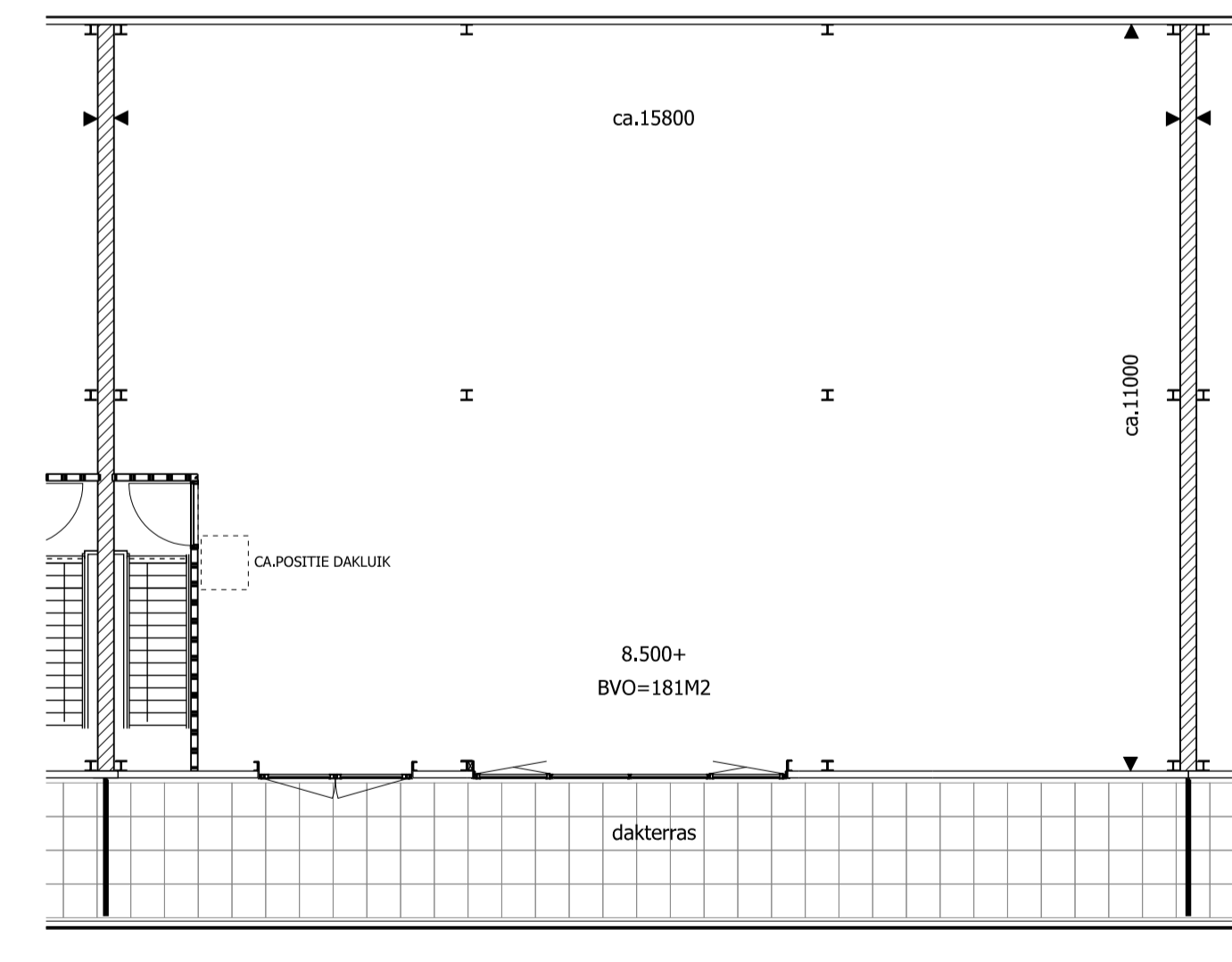
2e VERDIEPING UNIT BOUWNUMMER 27
