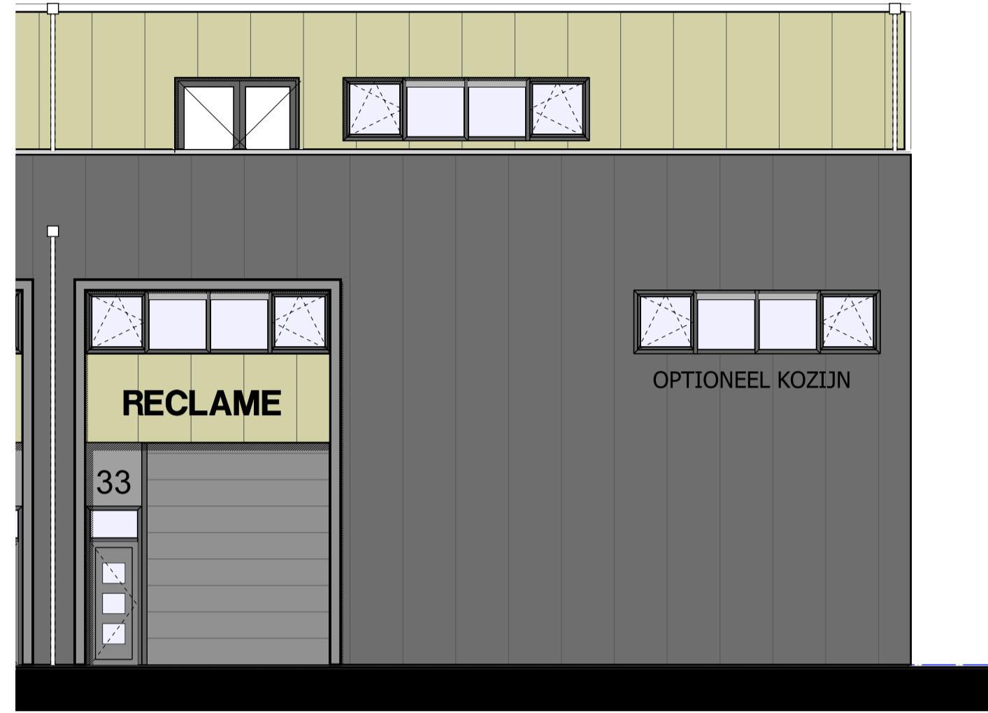
VOORAANZICHT UNIT BOUWNUMMER 33
