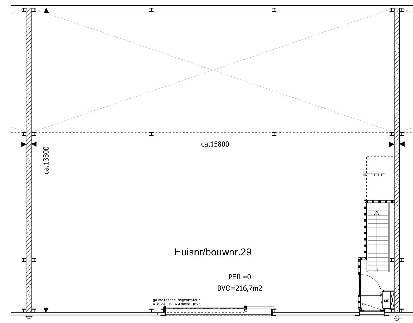
PLATTEGROND UNIT BOUWNUMMER 29
