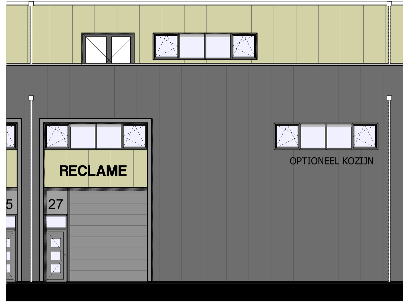
VOORAANZICHT UNIT BOUWNUMMER 27
