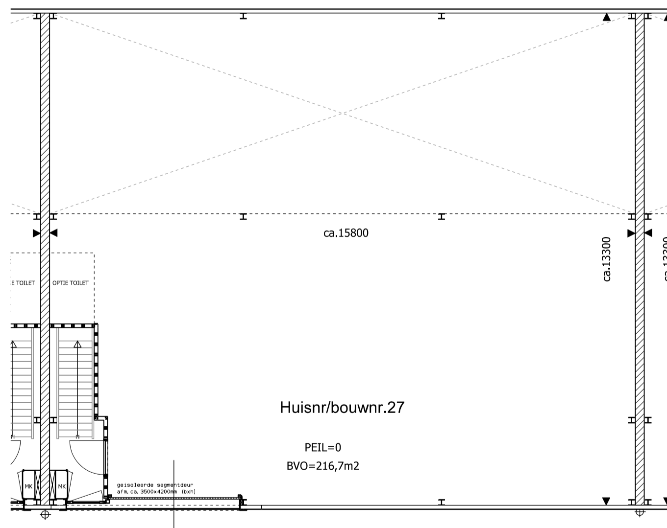
PLATTEGROND UNIT BOUWNUMMER 27
