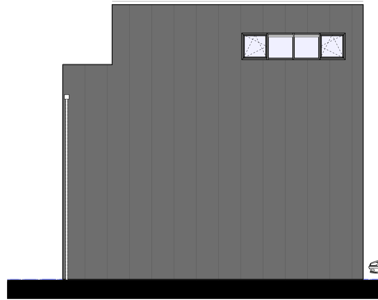
ZIJAANZICHT UNIT BOUWNUMMER 33
