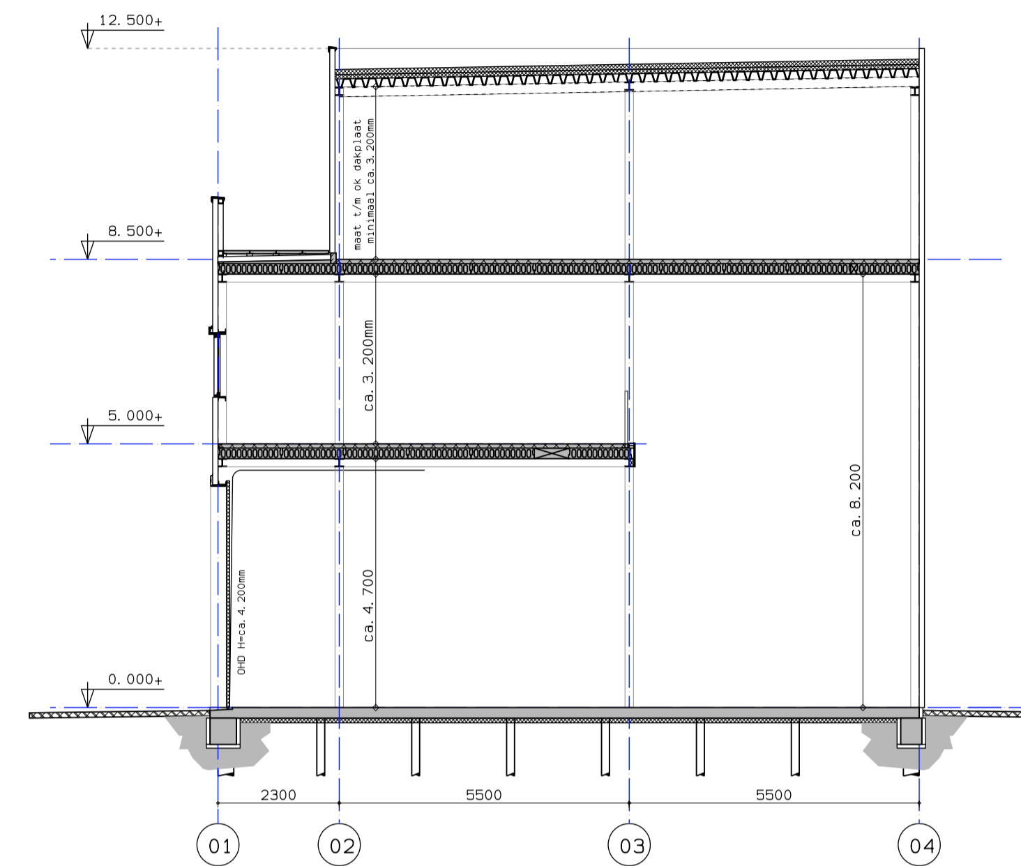
DWARSDOORSNEDE UNIT BOUWNUMMER 25
