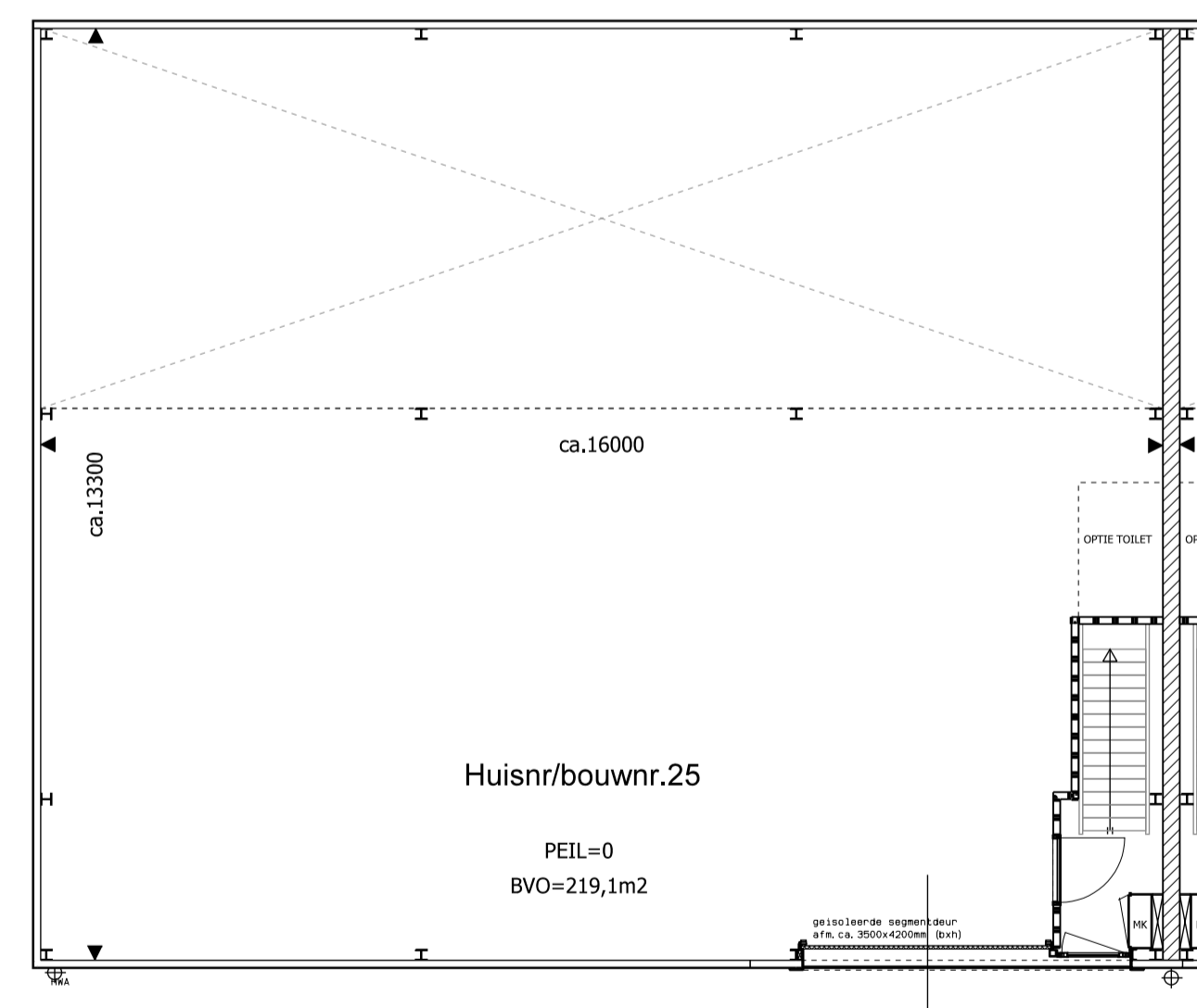
PLATTEGROND UNIT BOUWNUMMER 25
