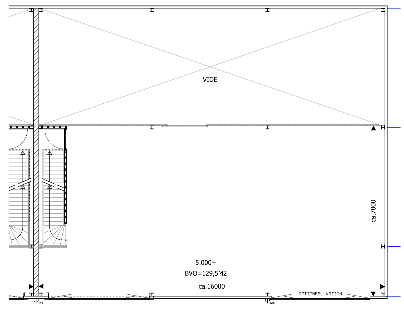
1e VERDIEPING UNIT BOUWNUMMER 33
