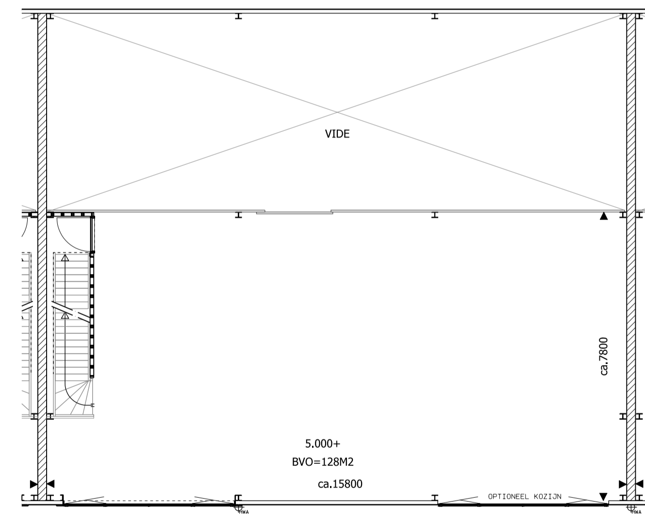
1e VERDIEPING UNIT BOUWNUMMER 27
