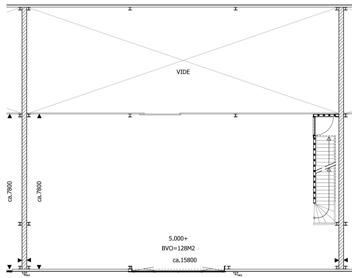
1e VERDIEPING UNIT BOUWNUMMER 29
